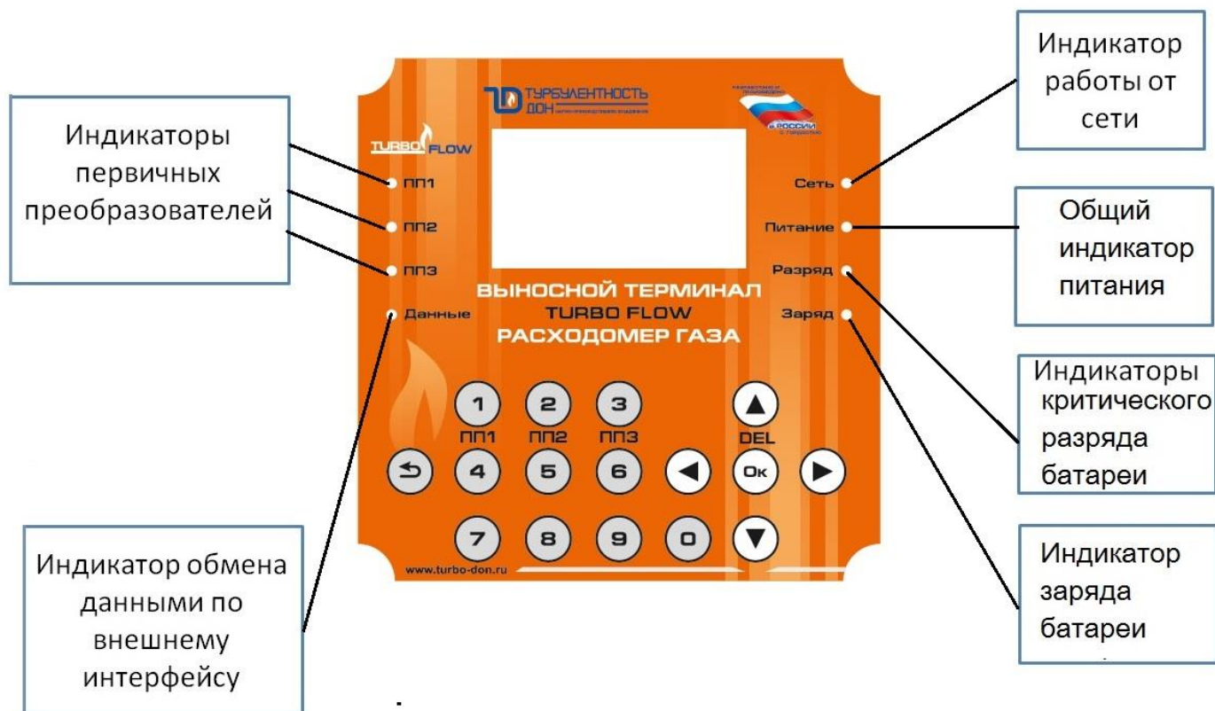
Рисунок 1 Внешний вид терминала
